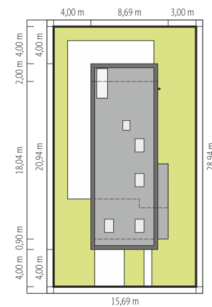
Schemat uwzględnia minimalne odległości od budynku do granicy działki. Szczegóły w zakładce: jak czytać projekt?
