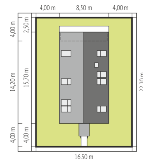
Schemat uwzględnia minimalne odległości od budynku do granicy działki. Szczegóły w zakładce: Jak czytać projekt?
