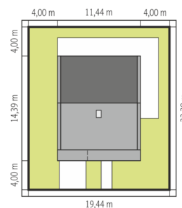
Schemat uwzględnia minimalne odległości od budynku do granicy działki. Szczegóły w zakładce: Jak czytać projekt?
