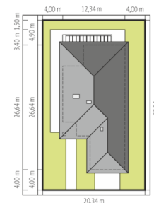
Schemat uwzględnia minimalne odległości od budynku do granicy działki. Szczegóły w załączniku: jak czytać projekt?
