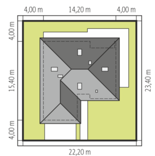
Schemat uwzględnia minimalne odległości od budynku do granicy działki. Szczegóły w zakładce: Jak czytać projekt?
