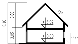
Schemat przekroju
